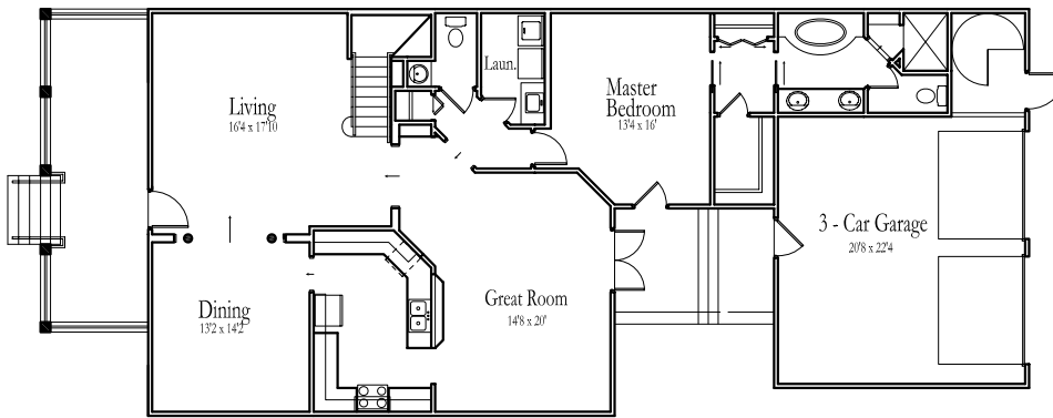
Floor Plan N.T.S
