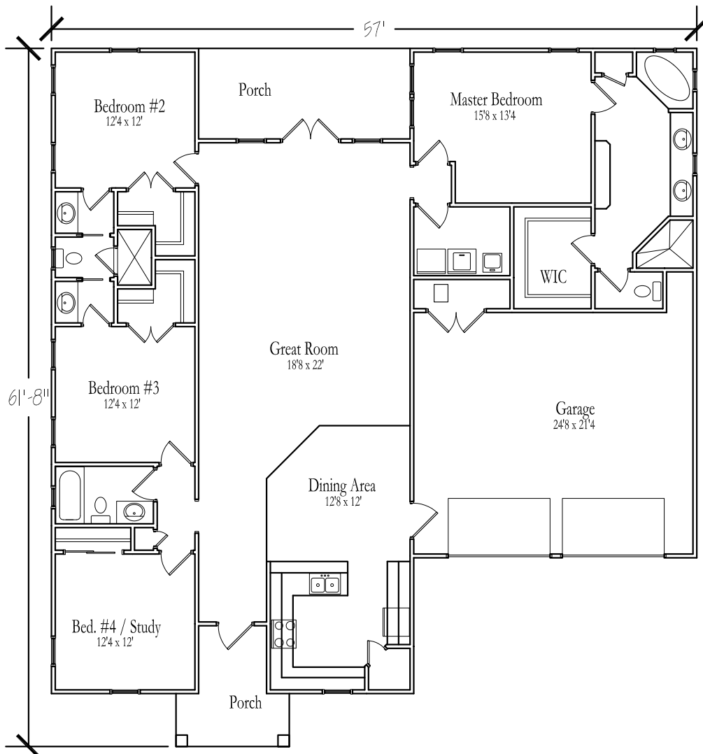
Floor Plan N.T.S
