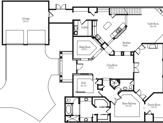
Floor Plan N.T.S
